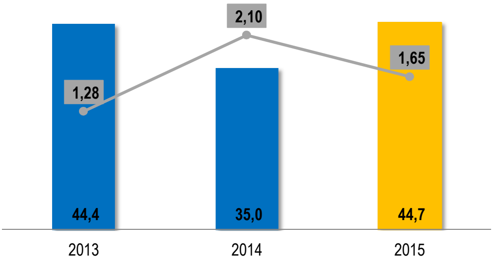
EBITDA
