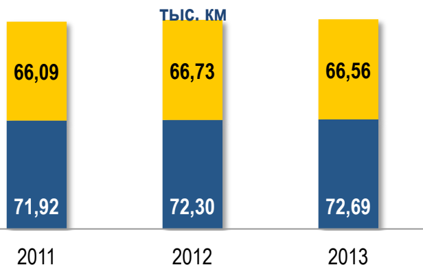
Протяженность линий электропередач, тыс. км
