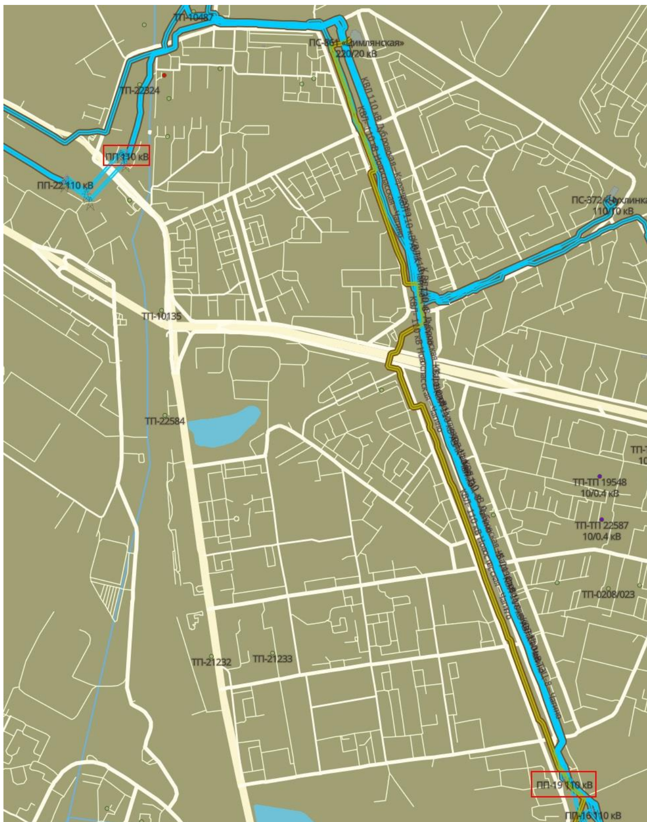
Рисунок 2. Ситуационный план КВЛ 110 кВ Чагино - АЗЛК I, II цепь.
