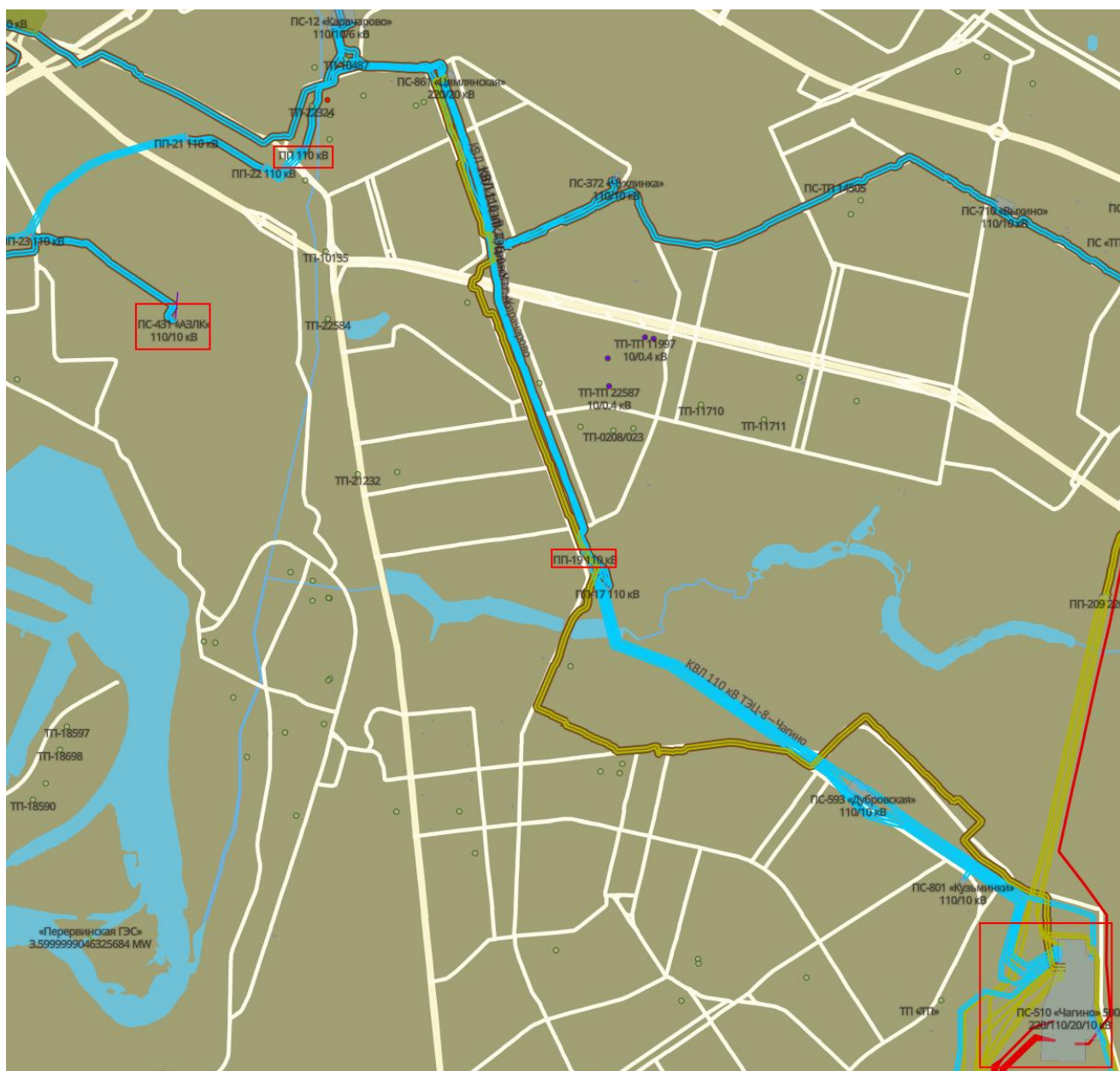
Рисунок 1. Общий план КВЛ 110 кВ Чагино - АЗЛК I, II цепь.
