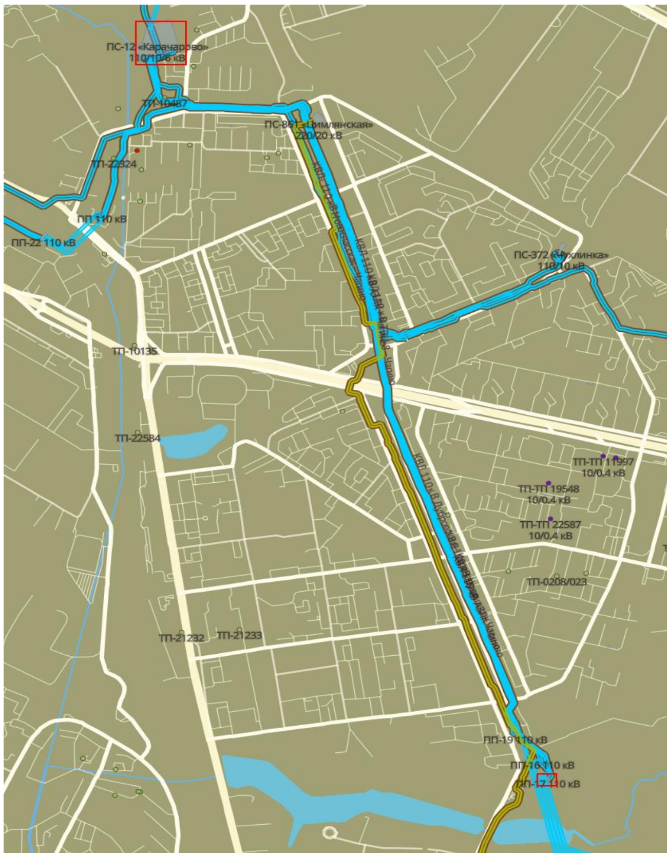
Схема 1. Ситуационный план КВЛ 110 кВ Дубровская - Карачарово I, II цепь
