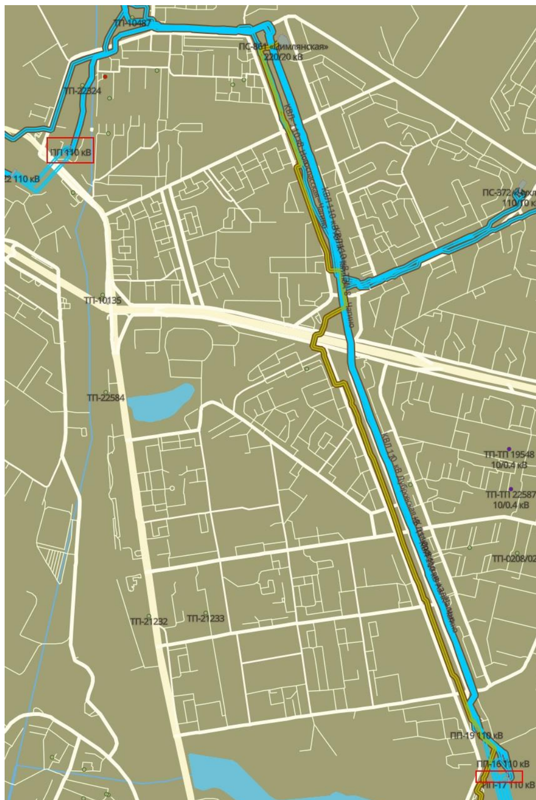
Рисунок 2. Ситуационный план КВЛ 110 кВ Чагино - Новоспасская.
