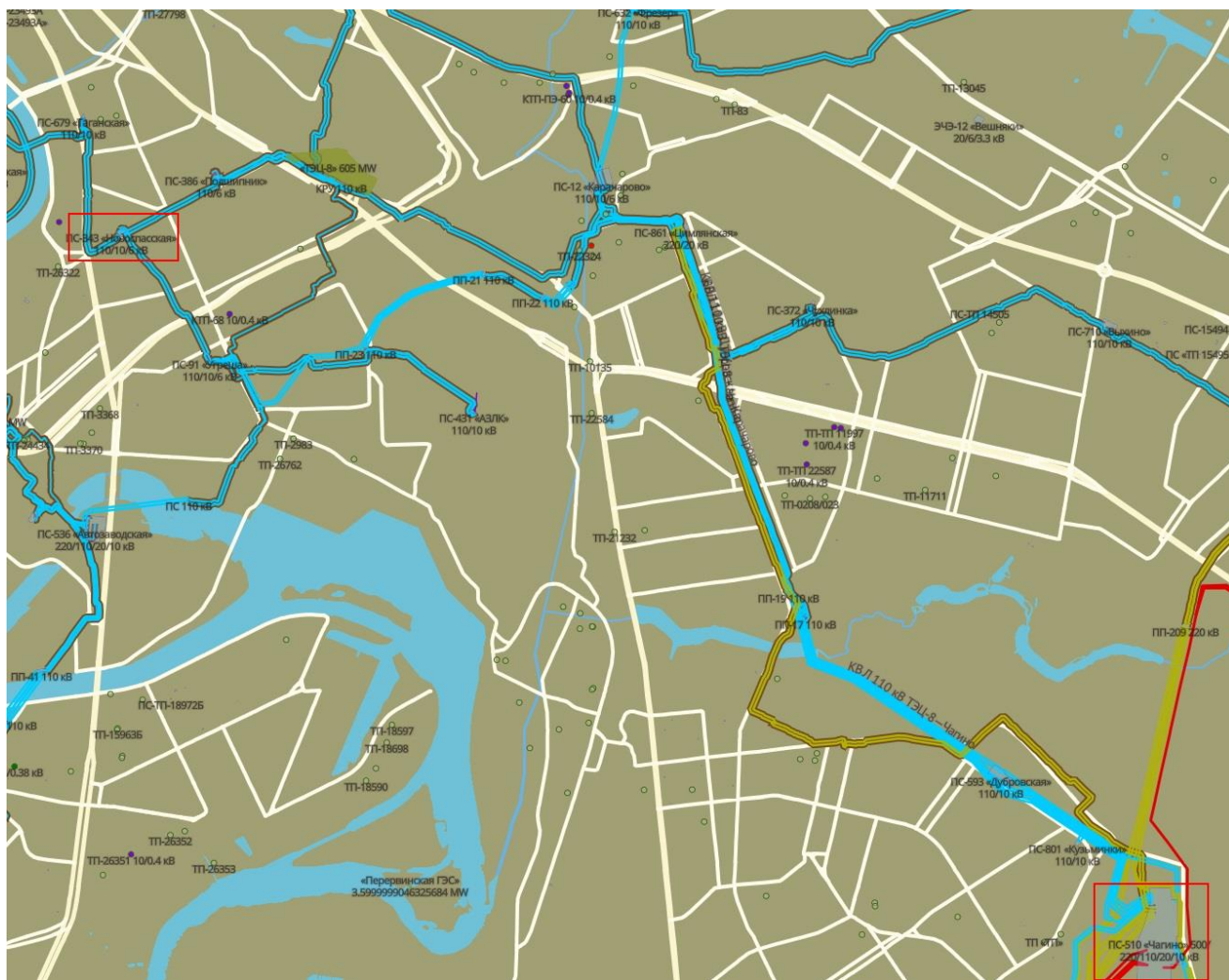
Рисунок 1. Общий план КВЛ 110 кВ Чагино - Новоспасская.
